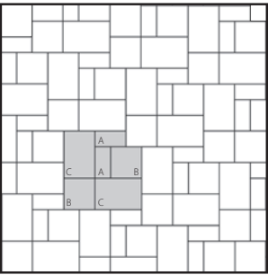
Patrón N.º 2 para unidades A, B y C A-33 % B-33 % C-33 %
