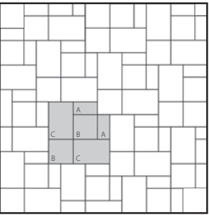
Patrón N.º 1 para unidades A, B y C A-33 % B-33 % C-33 %
