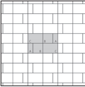
Patrón N.º 4 para unidades A, B y C A-33 % B-33 % C-33 %
